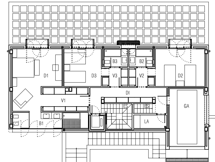
PLANTA PRIMERA / FIRST FLOOR 1 / 200
