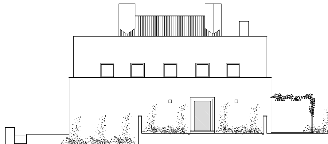
ALZADO A LA CALLE / STREET FACADE 1 / 200
