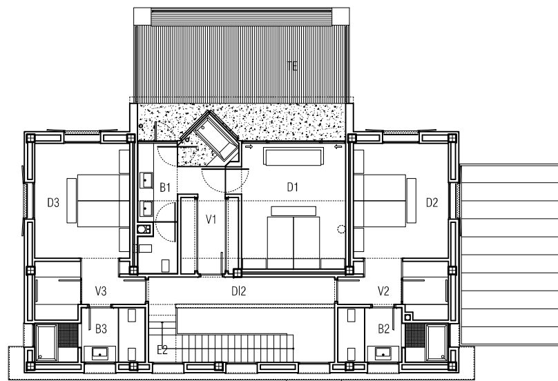
PLANTA PRIMERA / FIRST FLOOR 1 / 200
