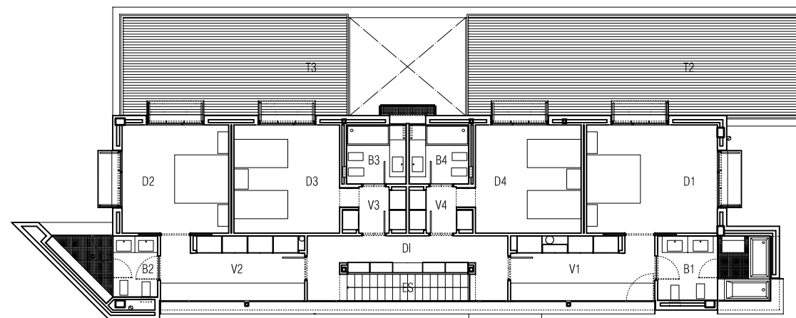
PLANTA PRIMERA / FIRST FLOOR 1 / 200
