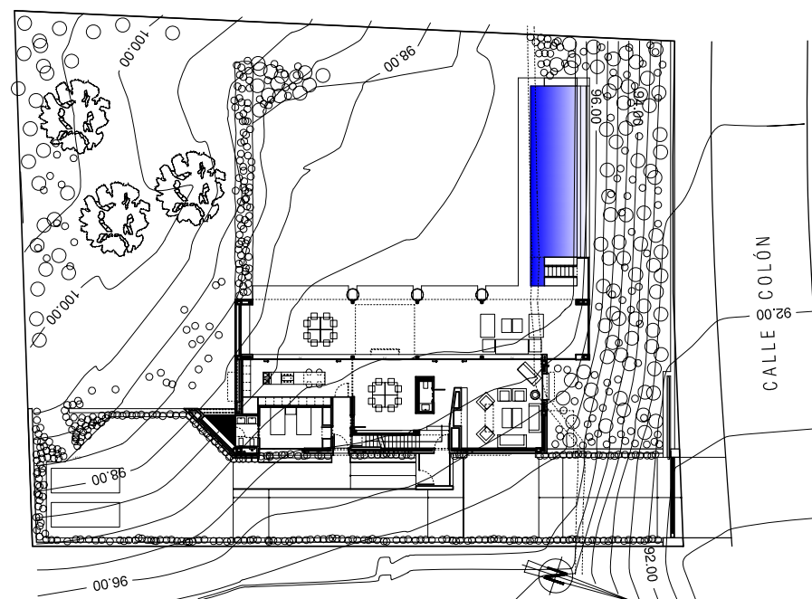
PLANTA DE ORDENACIÓN / PLOT PLAN 1 / 500
